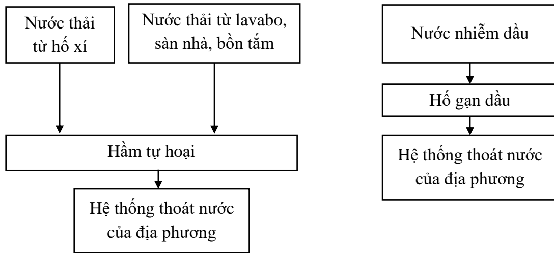
Hình 3. Sơ đồ thu gom và thoát nước thải tại cơ sở
